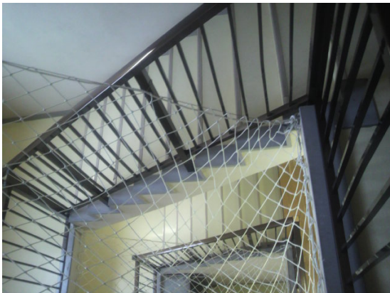
【階段転落防止ネット】
